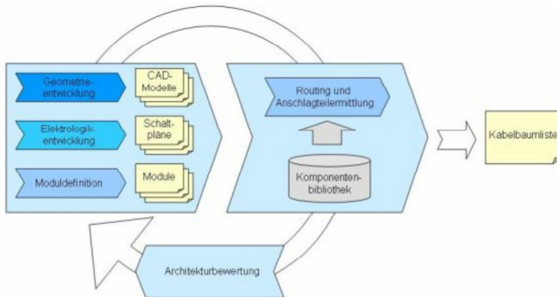
Abbildung 1: Kabelbaum-Entwicklungsprozess
