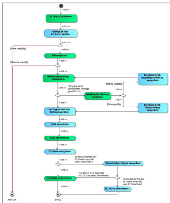
Modellierter Ablauf
