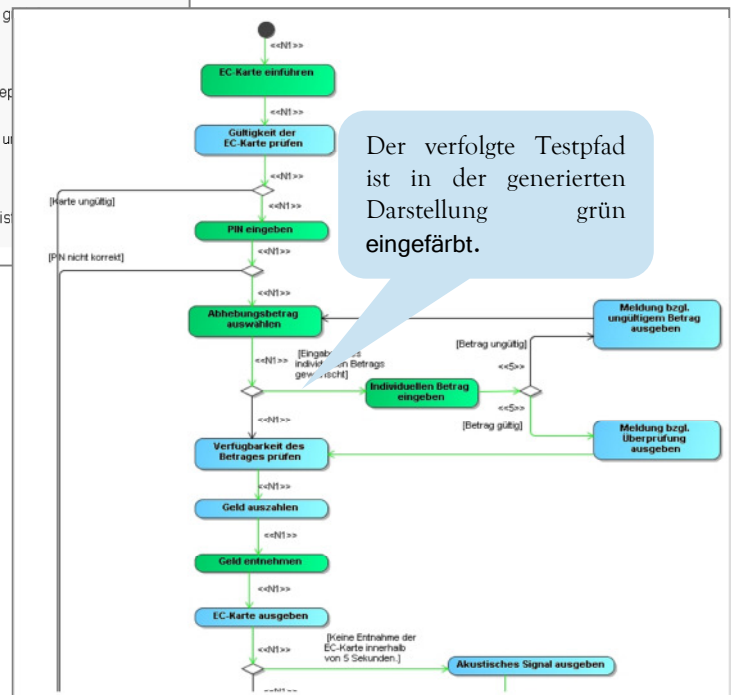
Visualisierung eines generierten Testfalls
